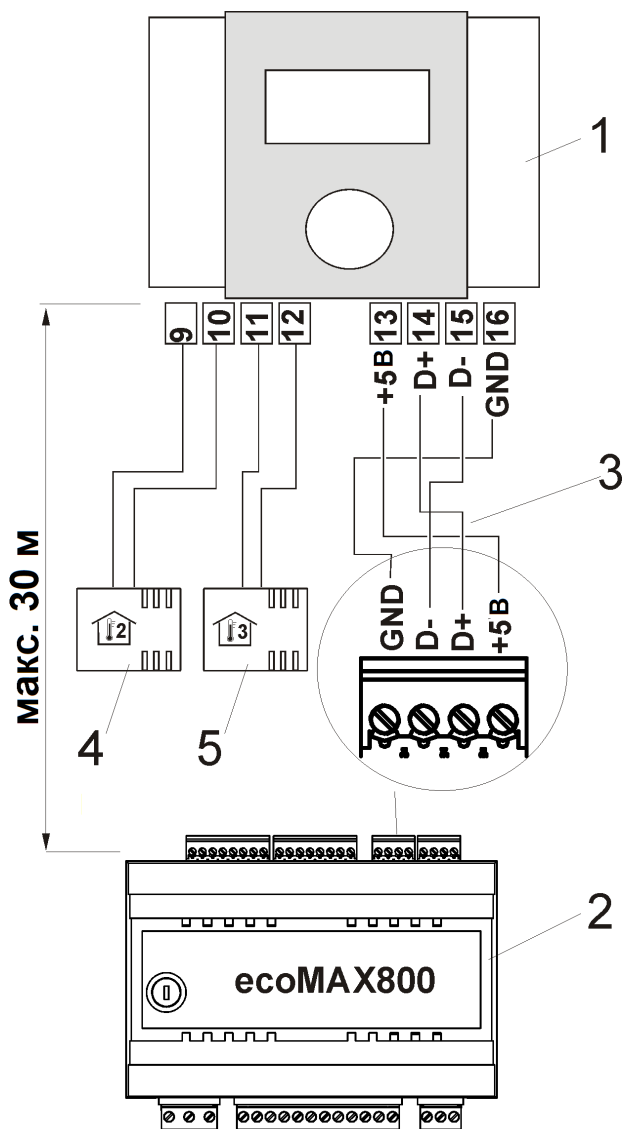
Рис. 8.3 Схема электрического соединения, где: 1 – комнатная панель ecoSTER200, 2 – регулятор ecoMAX800 R или T, 3 – соединительный провод, 4 – комнатный датчик термостата 2 тип СТ7, 5 – комнатный датчик термостата 3 тип СТ7.
