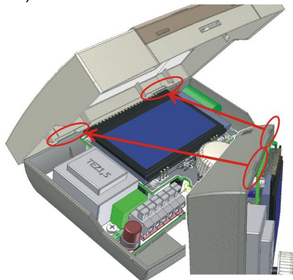
Рис. 8.5 Закрытие корпуса - шаг первый, (Смотровой чертеж)
