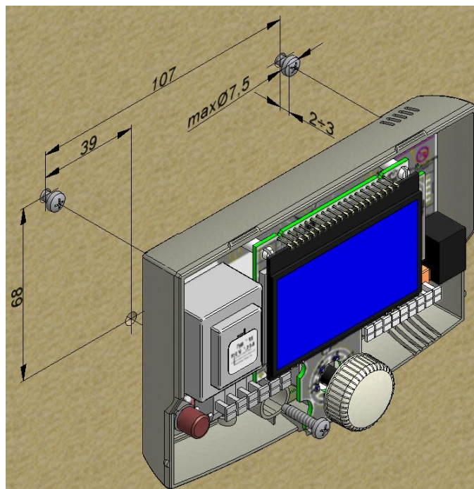
Рис. 8.2 Монтаж регулятора на стене (Справочный чертеж)
