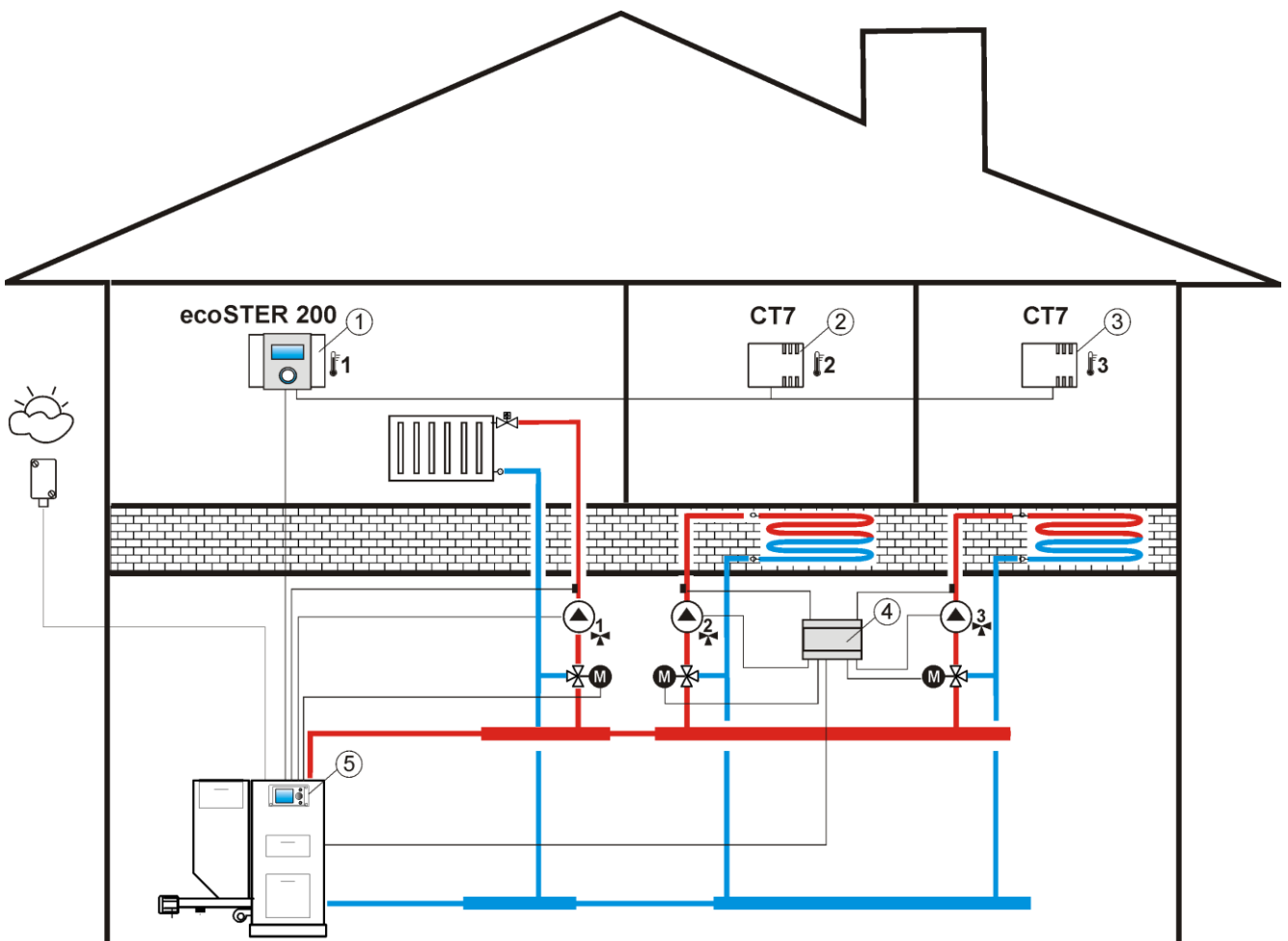
Рис. 8.7 2 Схема взаимодействия ecoSTER с ecoMAX800, где: 1 – ecoSTER200, 2- комнатный датчик термостата 2 тип CT7, 3- комнатный датчик термостата 3 тип CT7, 4- модуль MX.01 (расширяет систему на 2 нагревательных контура), 5 - регулятор ecoMAX800R или T.
